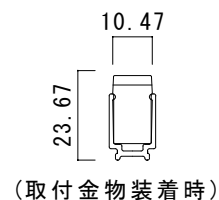
灯具本体部分断面 (A-A' 部断面)
