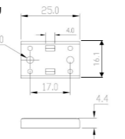
器具取付金物
